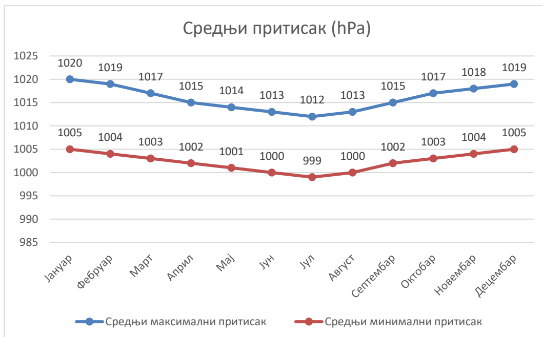
Графикон 4: Средњи просечни минимални и максимални притисак по месецима
