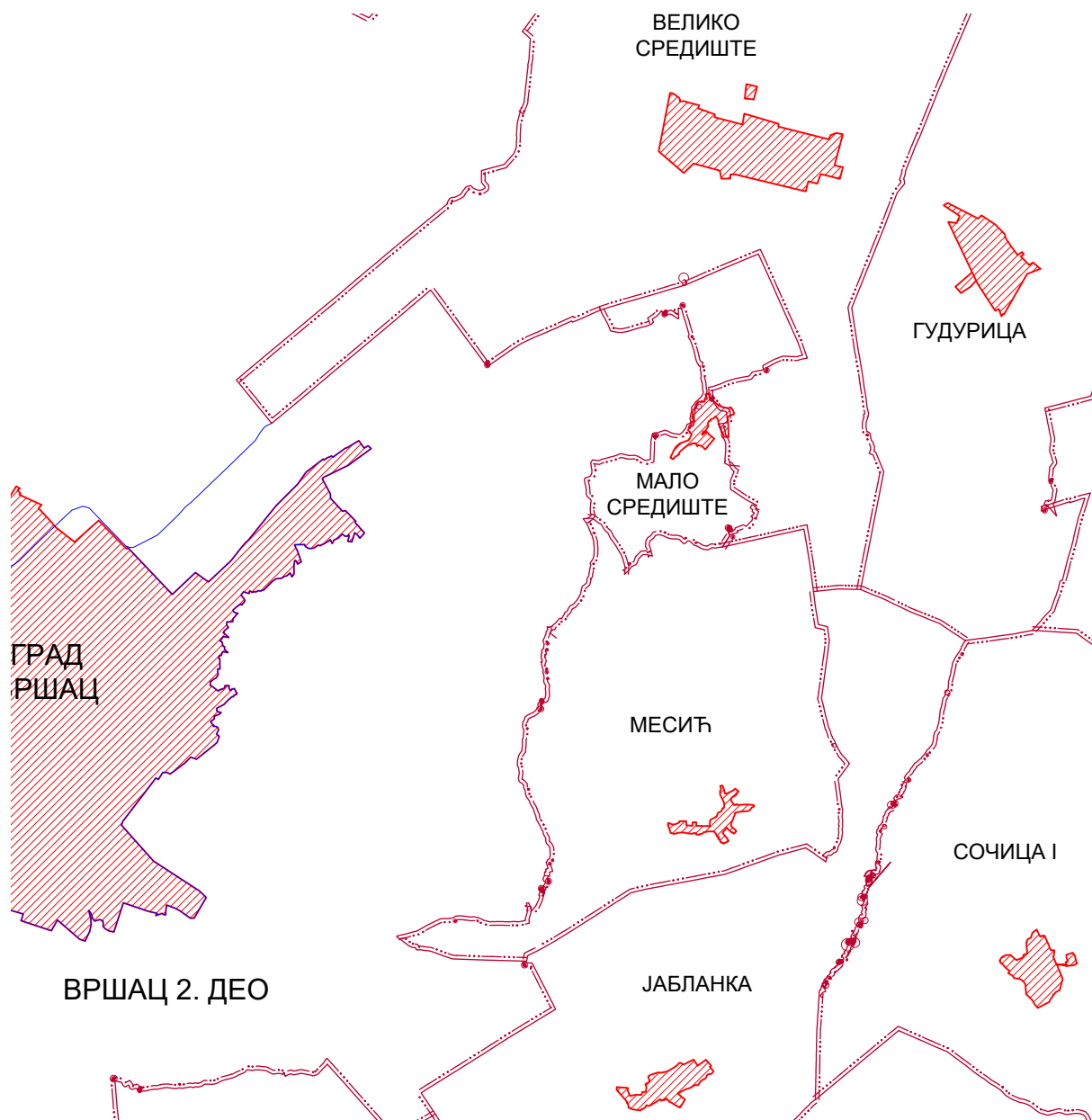
Слика: Подручје града Вршца и положај катастарских општине Месић
