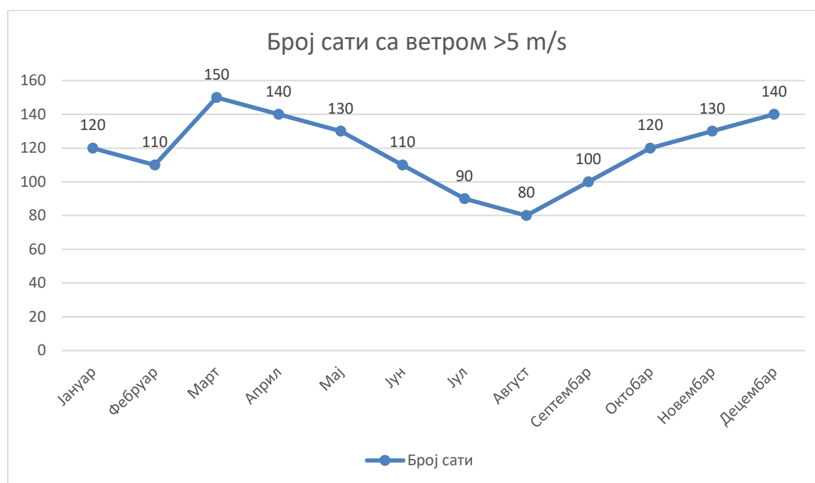
Графикон 6: Статистика ветровитих дана на месечном нивоу (број сати са ветром >5 m/s)
