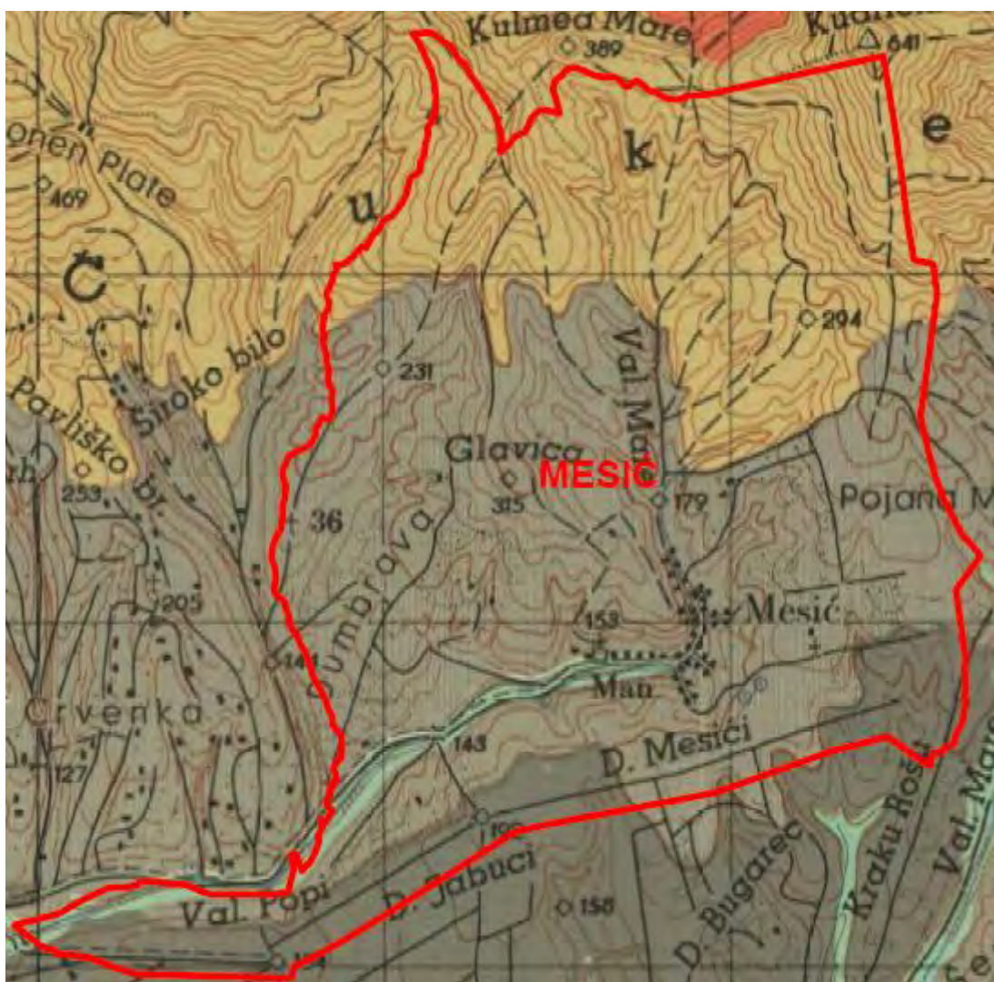
Слика 7: Педолошка карта КО Месић
