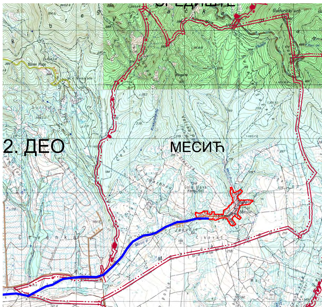
Слика 2: Мрежа водотокова и канала на КО Месић
