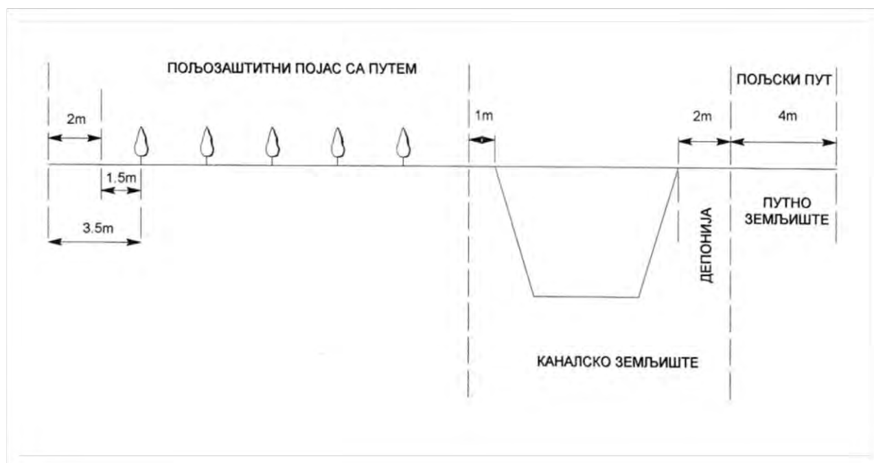
Слика 19: Пример профила пољозаштитног појаса са пољским путем и каналом
