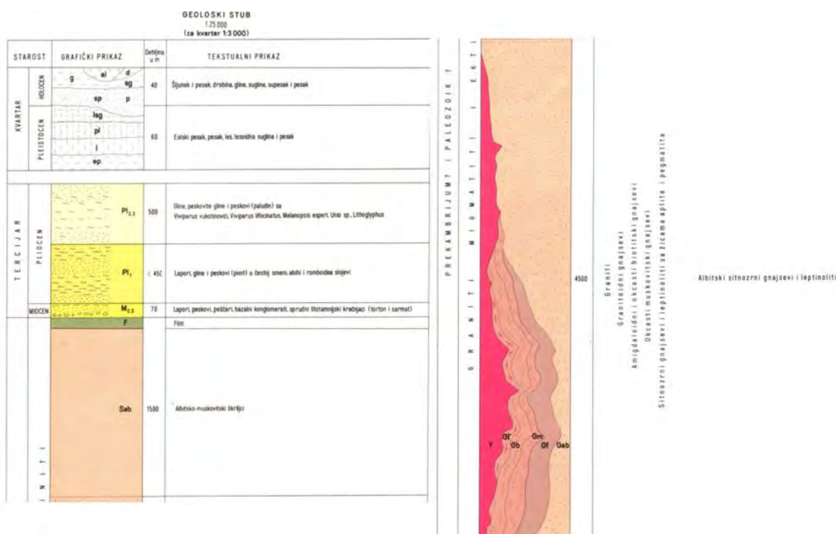
Слика 6: Геолошки стуб КО Месић
