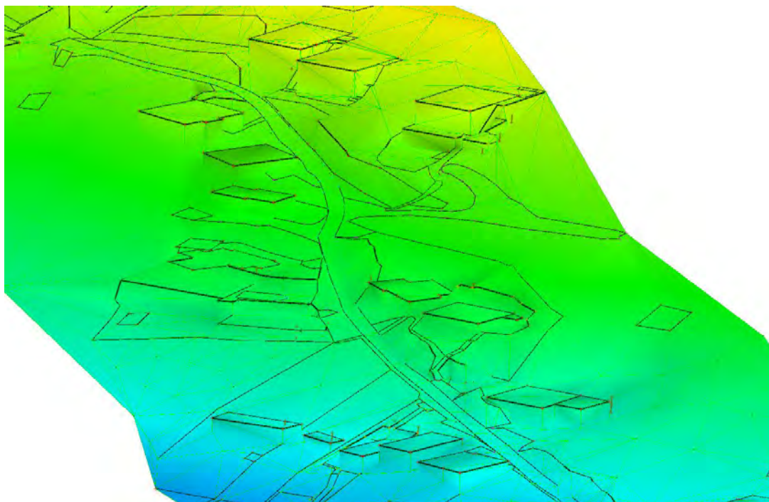
Слика 16: Изглед 3Д топографске подлоге и 3Д модела терена топографске подлоге
