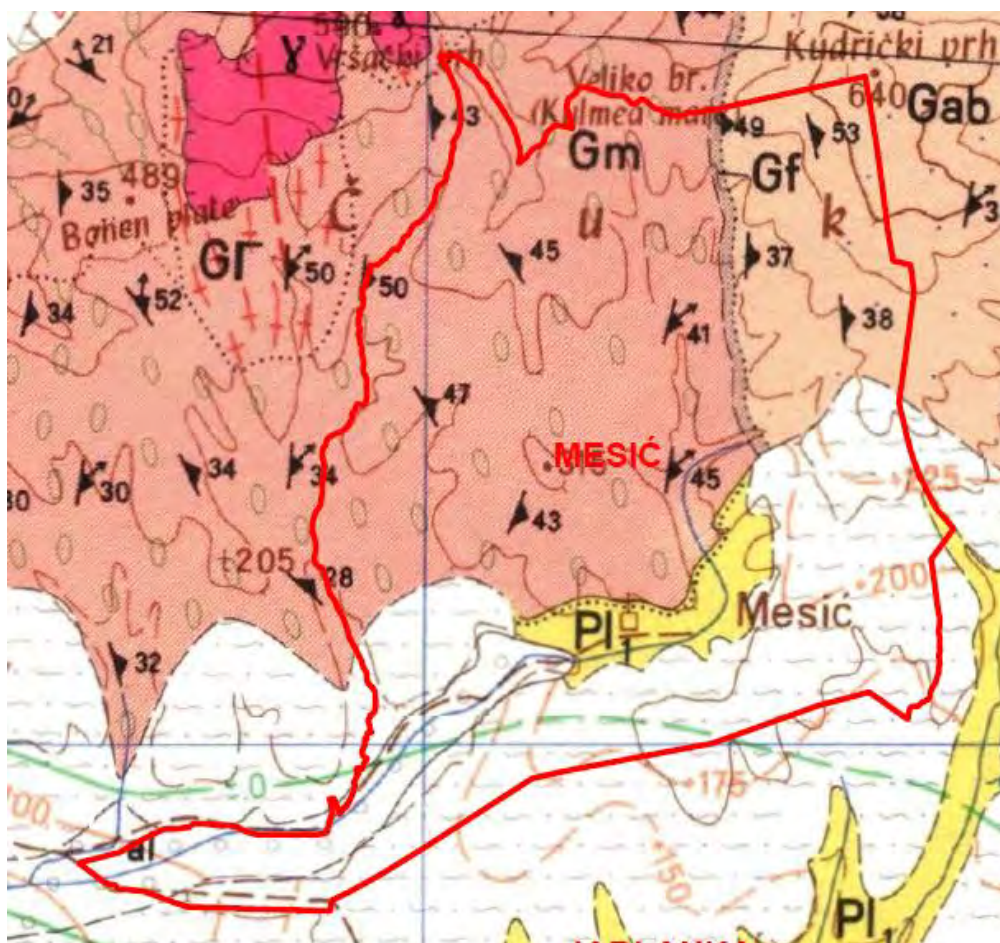
Слика 4: Геолошка карта КО Месић
